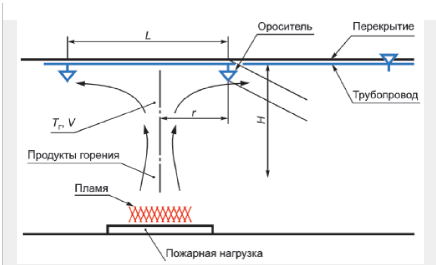
Рисунок В.1 - Расчетная схема
